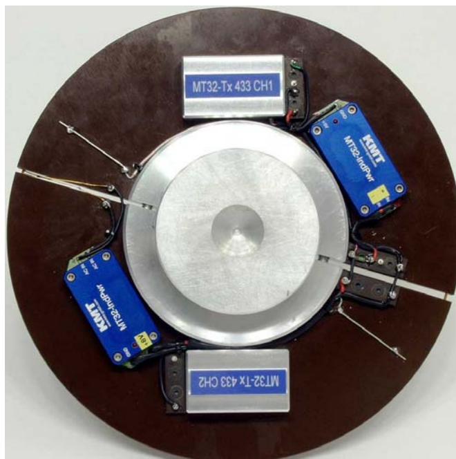
2-Kanal Scheiben-Telemetrie für Verseilmaschinen, zur Übertragung von TTL-Steuersignalen
