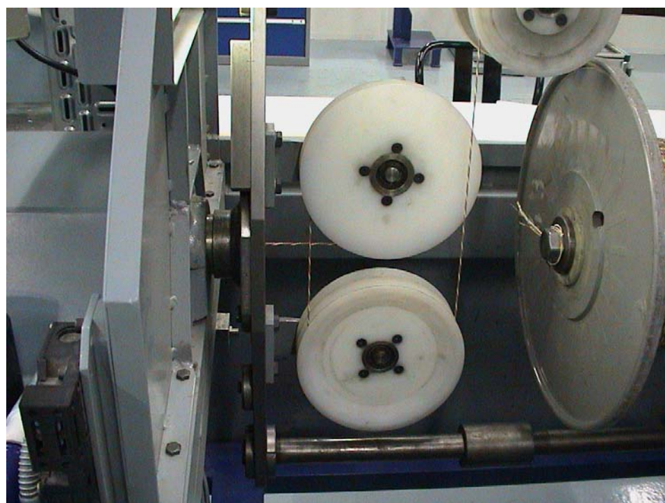
Verseilmaschine
