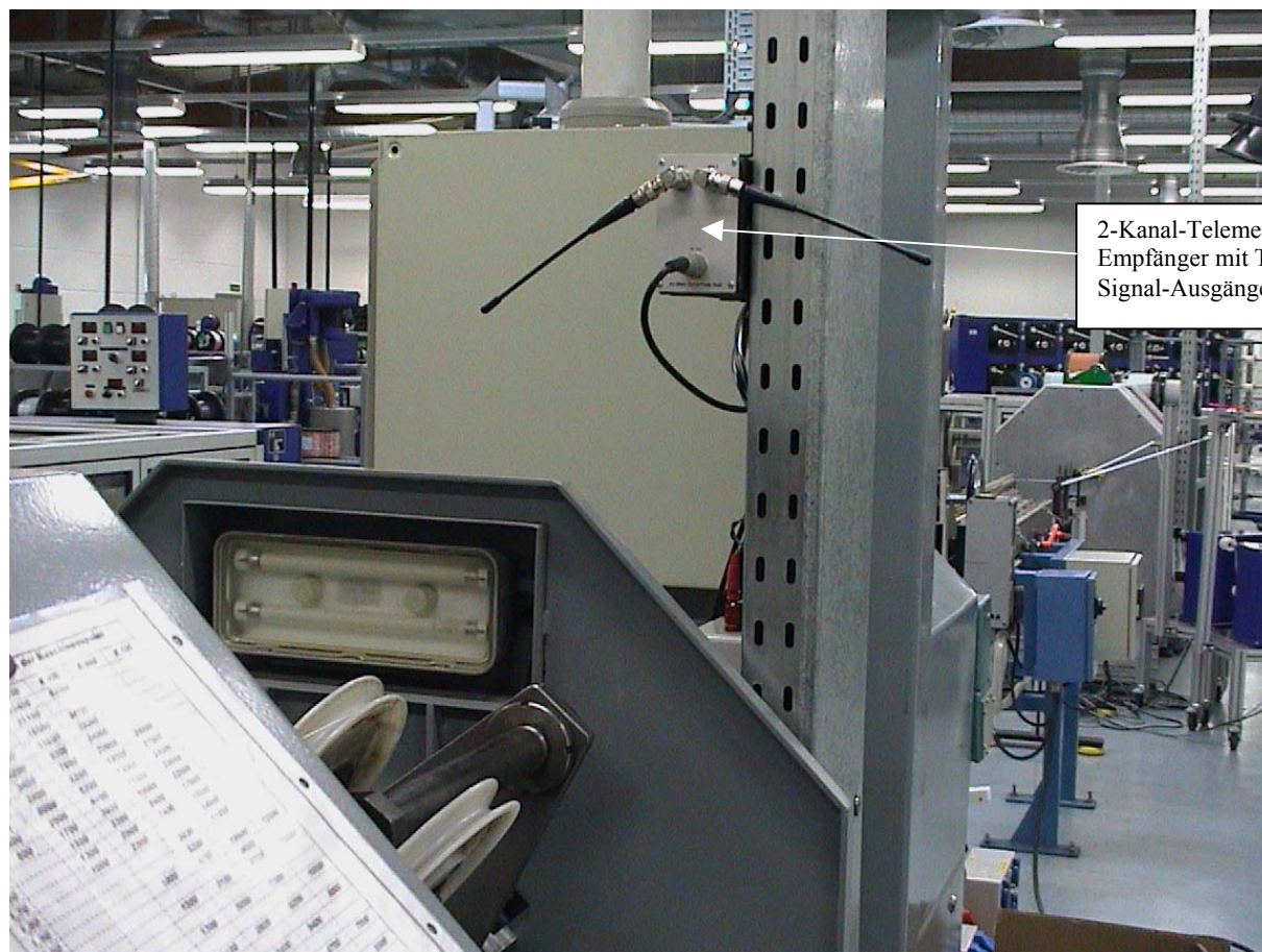
Verseilmaschine
